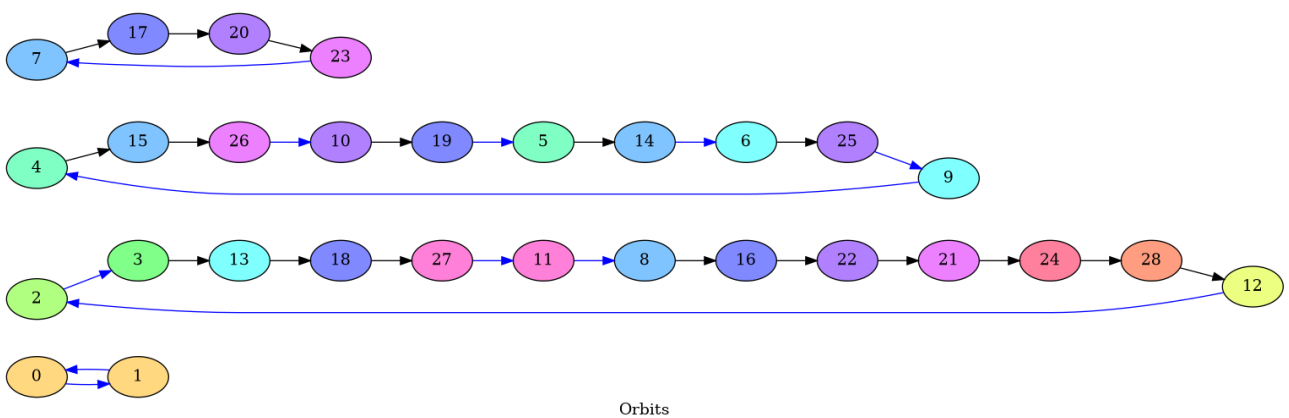
Fig. 6 \nu -orbits
